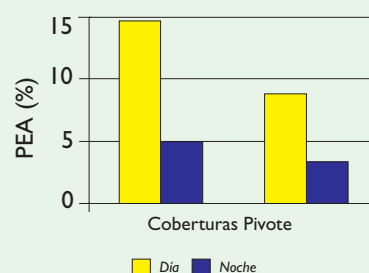
Figura 5. Valores medios de la pérdidas de evaporación y arrastre por el viento (PEA) en las evaluaciones de riegos diurnos y nocturnos en el prototipo de máquina de riego por aspersión (Pivote) y las coberturas fijas (Coberturas) de la finca del CITA en Montañana, Zaragoza.
