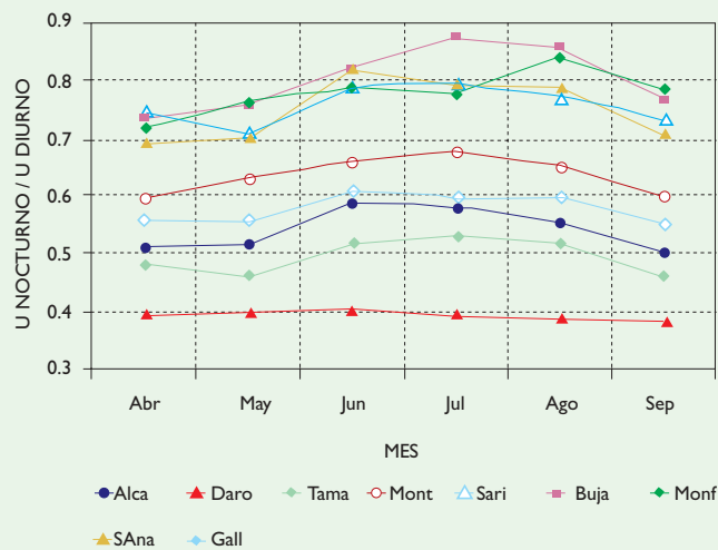
Figura 2. Cocientes entre las medias mensuales (abril a septiembre) para un año medio de la velocidad nocturna ( U nocturno) y la velocidad diurna ( U diurno) del viento a 2 m. Alca, Alcañiz; Daro, Daroca; Tama, Tamarite; Mont, Montañana; Sari, Sariñena; Buja, Bujaraloz; Monf, Monflorite; SAna, Santa Anastasia; Gall, Gallo-canta.
