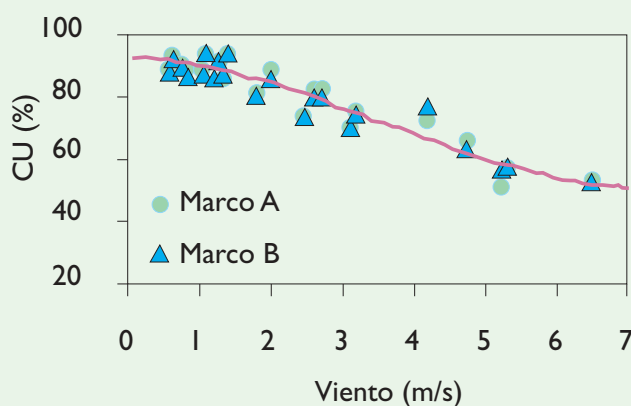
Figura 3. Relación entre el Coeficiente de Uniformidad (CU) y la velocidad del viento en dos marcos de aspersores de una cobertura fija instalada en marco cuadrado de 15 m x 15 m en la finca experimental del CITA en Montañana, Zaragoza.
